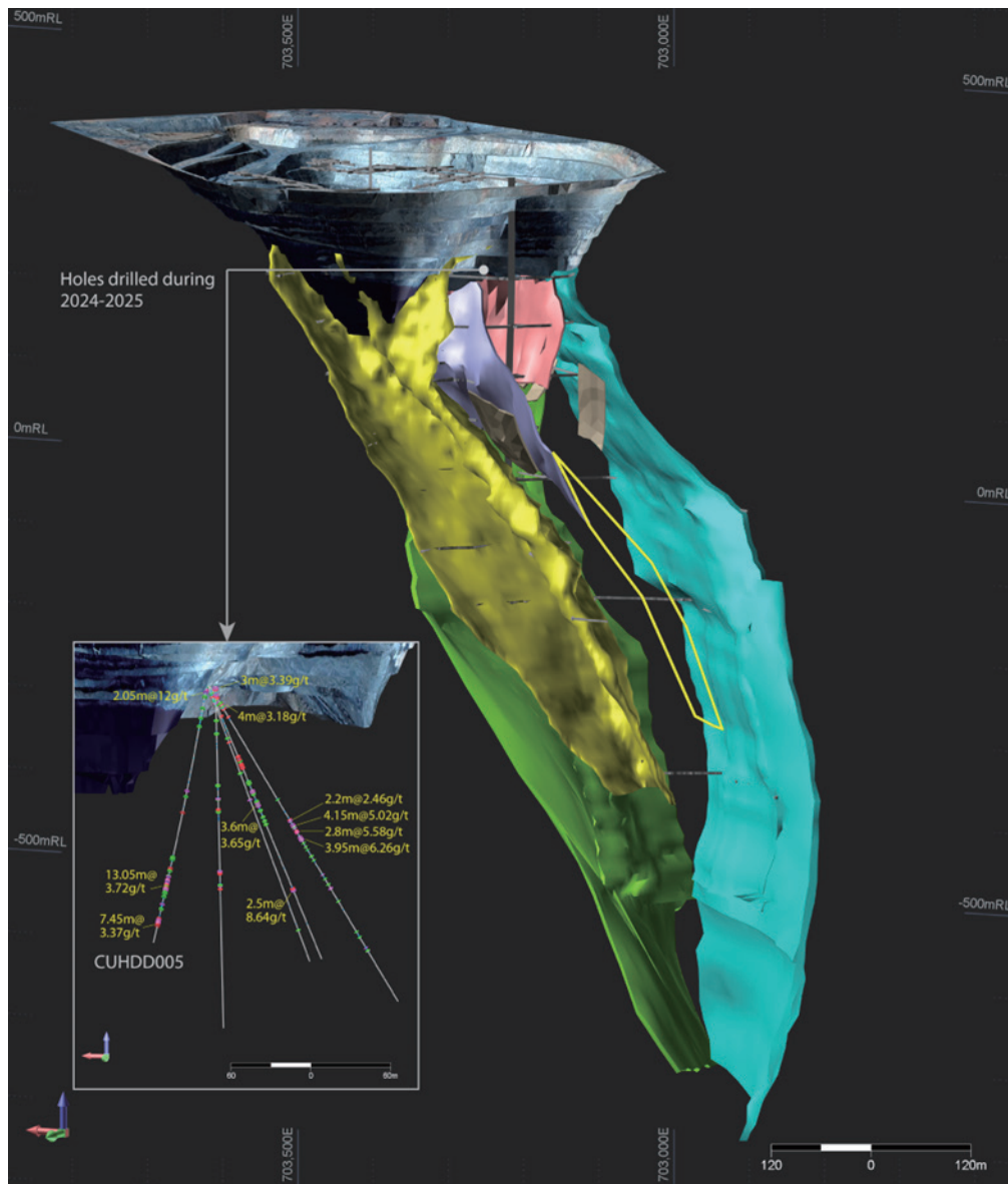
圖 2：Copperhead 金礦床之礦體分佈圖，顯示位於右側、以藍色標示的南部大型礦體尚未納入礦山設計；為優化礦山設計，該礦體適合採用地下扇形鑽探方式進行進一步勘探。
