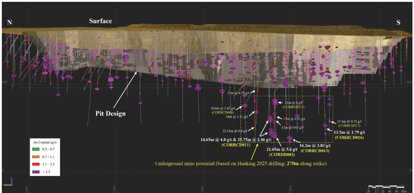
圖 1：Corinthia 金礦床之長剖面圖，顯示多條高品位金礦脈自地表向下延伸超過 300 米，其沿走向長度超過 270 米，且仍具進一步增長的潛力。
