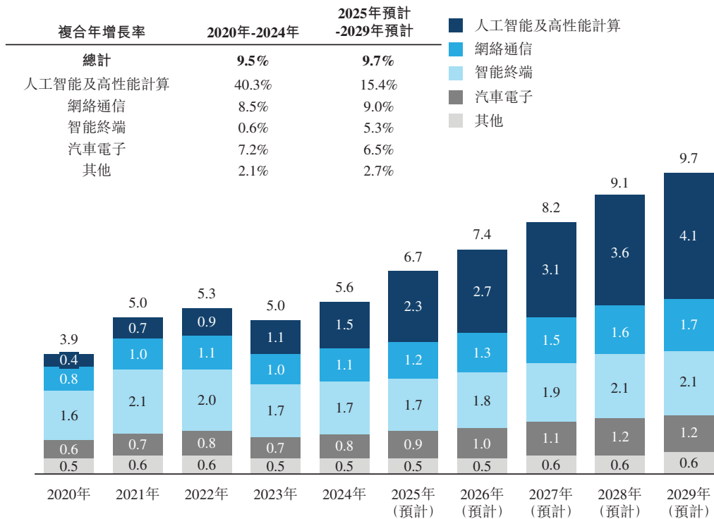
全球14層及以上高多層PCB市場規模，按應用領域劃分 (十億美元，2020-2029年預計)
