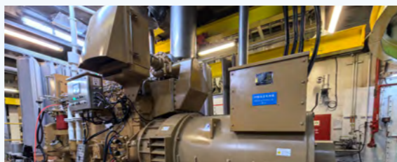
发电机组升级改造
