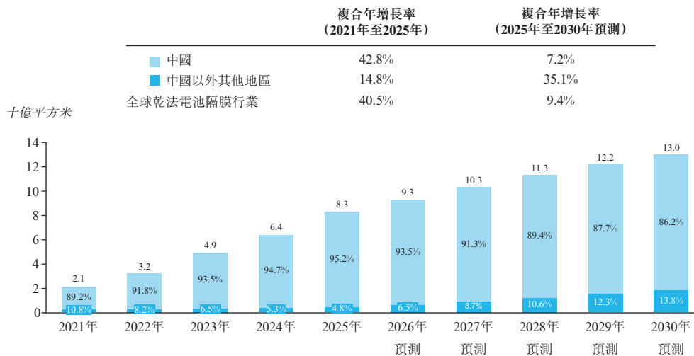
全球乾法電池隔膜行業(按出貨量計，2021年至2030年預測)
