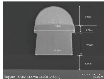
具有 18\mu\text{m} 凸點尺寸的Bumping
