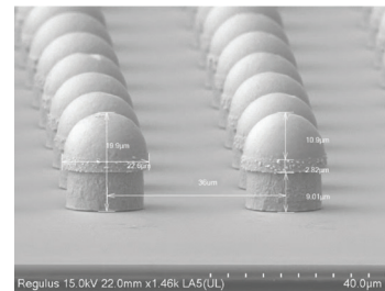
具有 36\mu\text{m} 凸點中心距的Bumping
